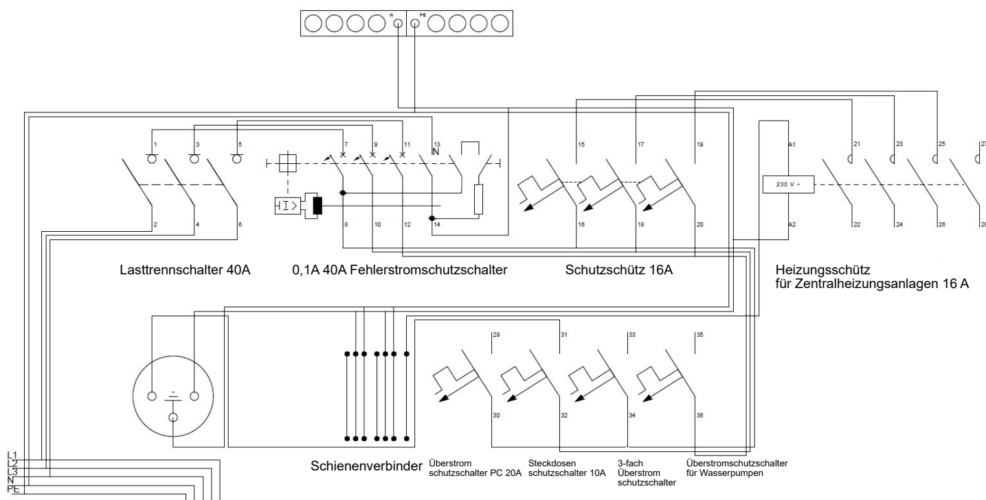
Abb. 8 Elektrischer Anschlusschema
